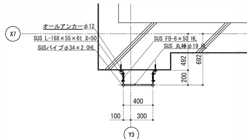
B断面図 S:1/15
