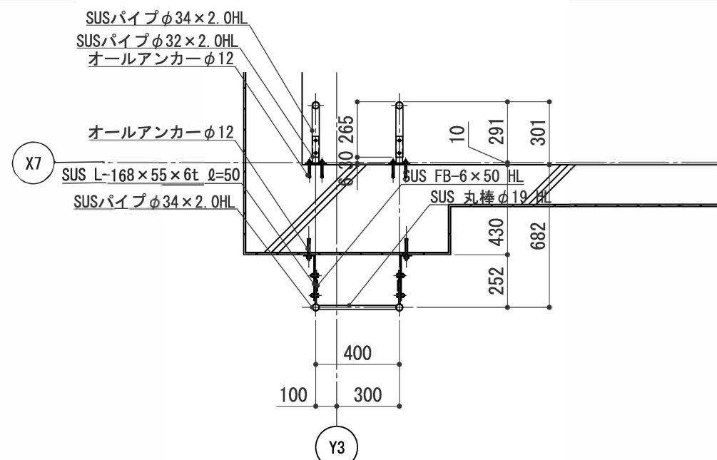
A断面図 S:1/15
