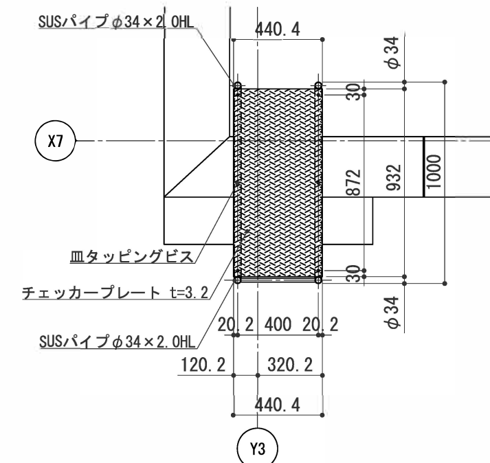
C断面図 S:1/15
